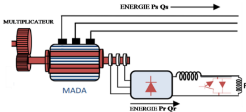
Fig. I. 12 : MADA à énergie rotorique dissipée [10].
