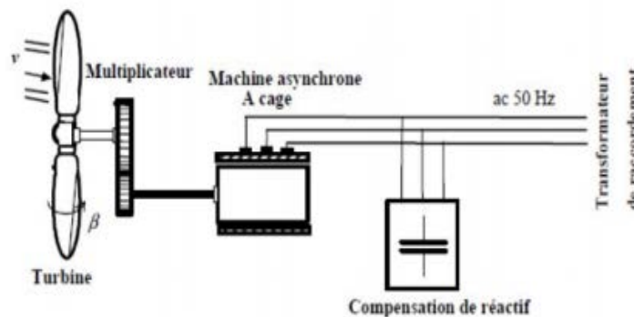
Fig. I. 6: Eolienne à vitesse fixe. [8]
