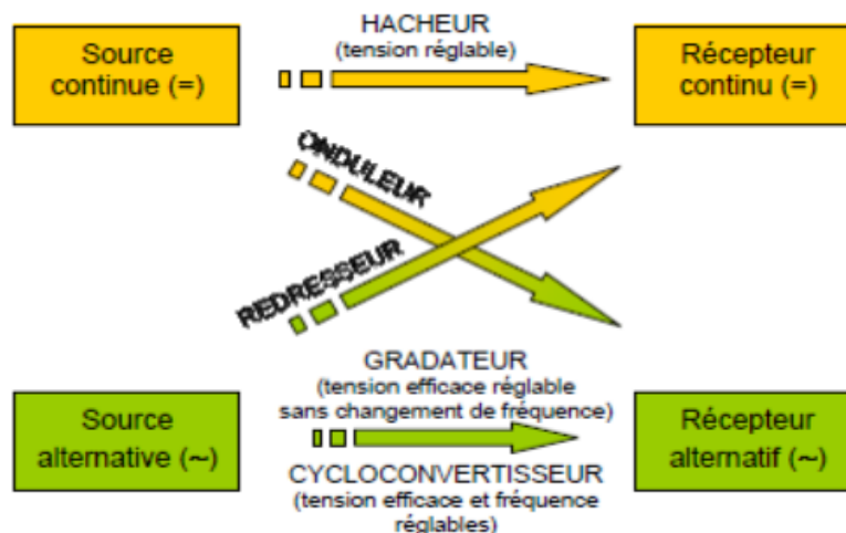
Fig. III 1:Famille des convertisseurs statiques [2].
